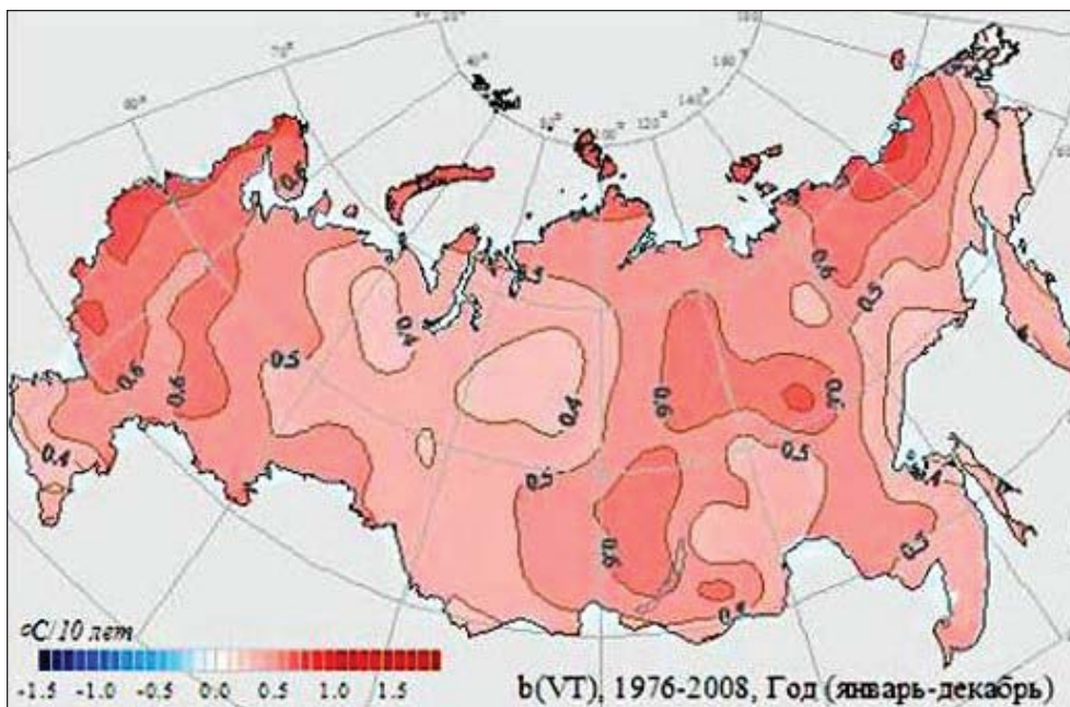
Рис. 2. Средняя скорость изменения среднегодовой температуры приземного воздуха на территории России по данным наблюдений за 1976-2008 гг. (в °C/10 лет). По материалам «Оценочного доклада об изменениях климата и их последствиях на территории Российской Федерации». Т.1 (2010:38).
