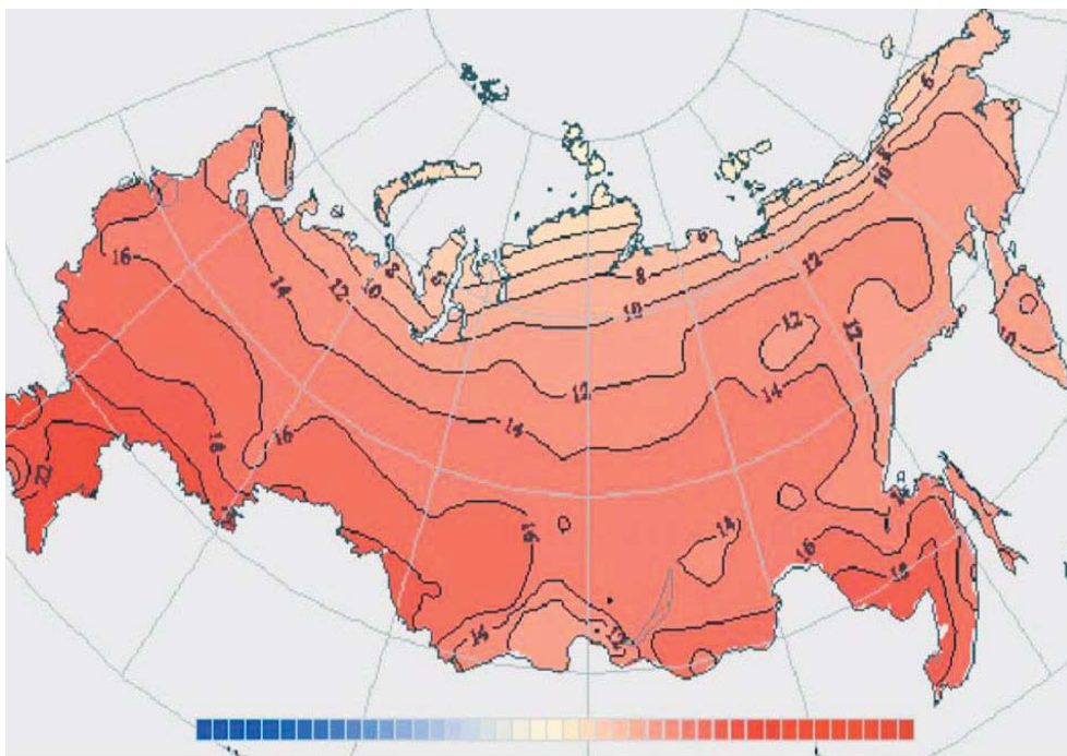
Рис.27. Средняя летняя температура приземного воздуха ( ^{\circ}\text{C} ) России за период 1961-1990гг. (цит. по ОД, том 1, 2008:12)
